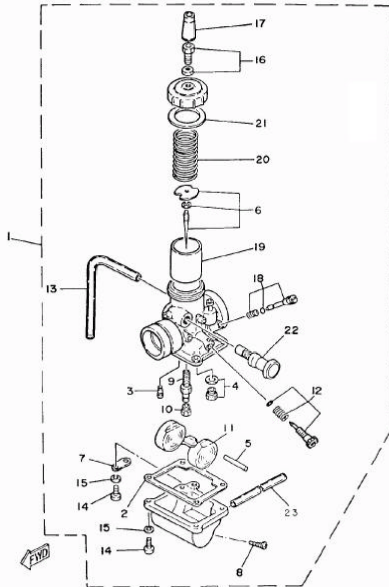
FIG. 05 - CARBURADOR
